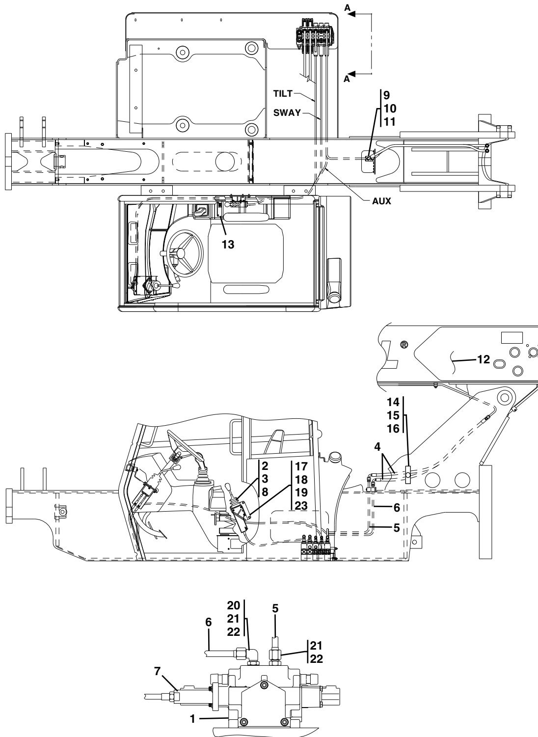
VIEW A-A
