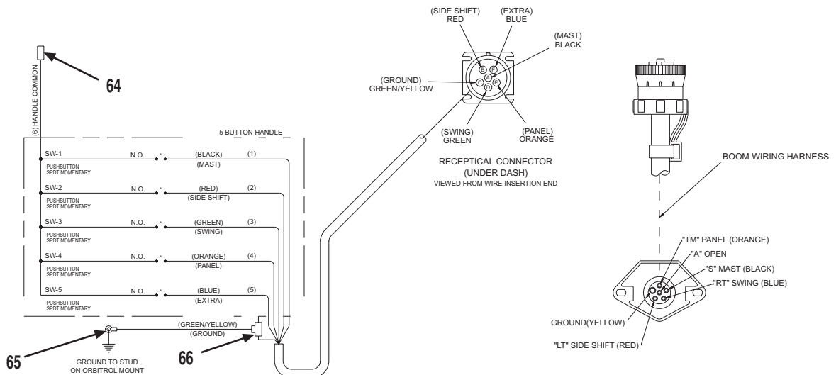
VIEW A-A
