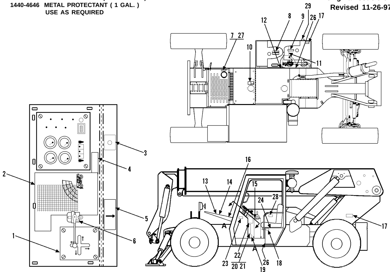
VIEW A-A
