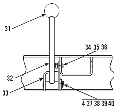
VIEW A-A
