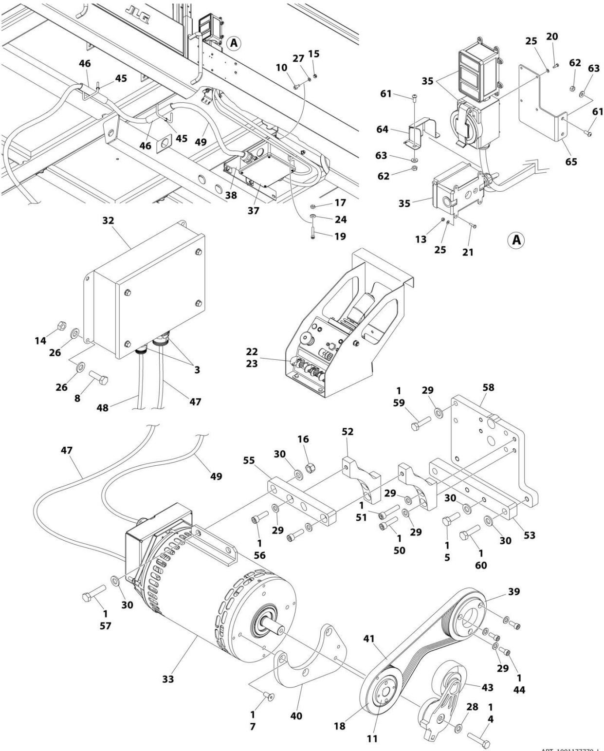
FIGURE 3-24. GENERATOR INSTALLATION - 4000W (KUBOTA DIESEL T4F)
