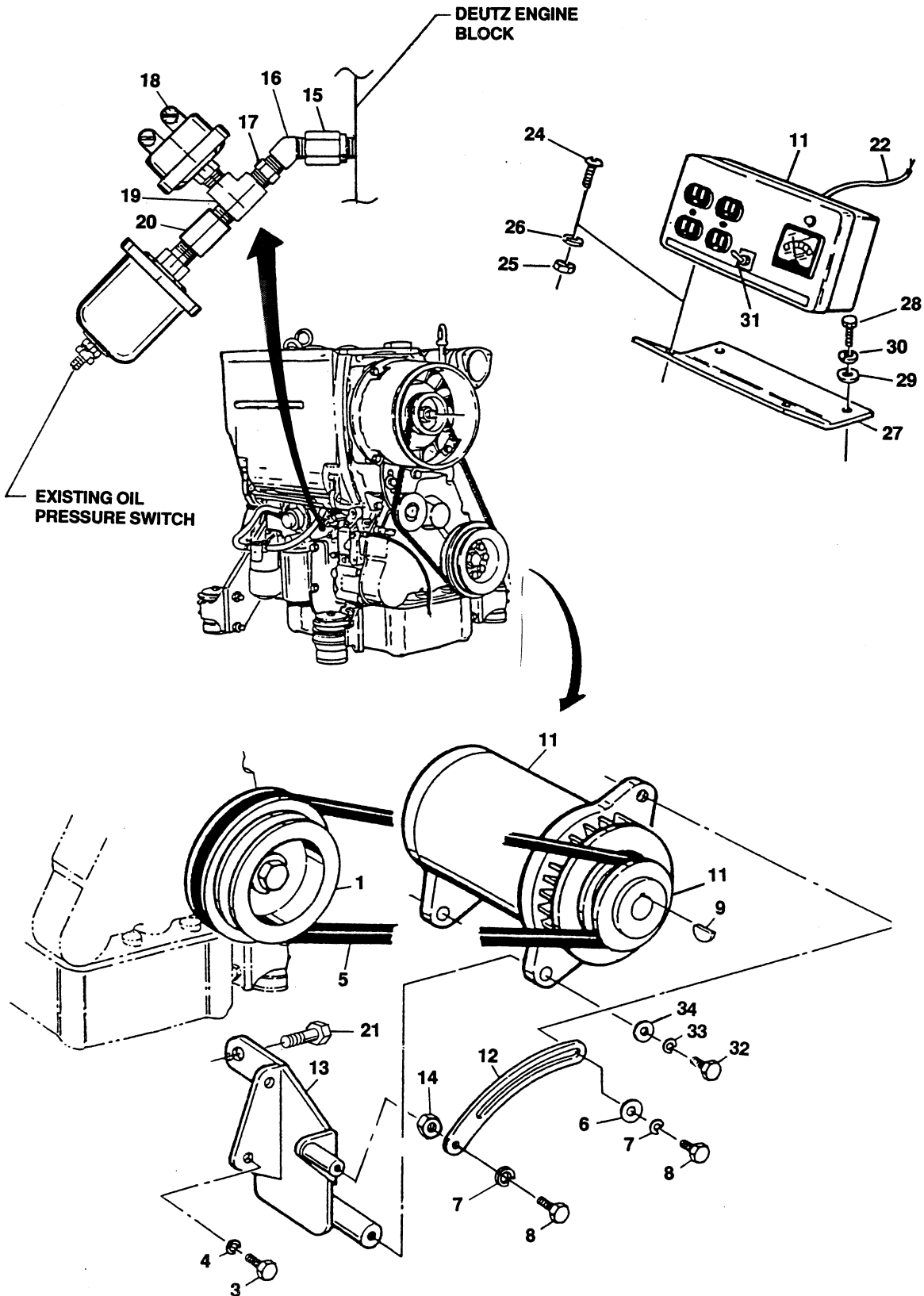
FIGURE 2-11. 110 VOLT GENERATOR INSTALLATION (DEUTZ) (OPTIONAL).
