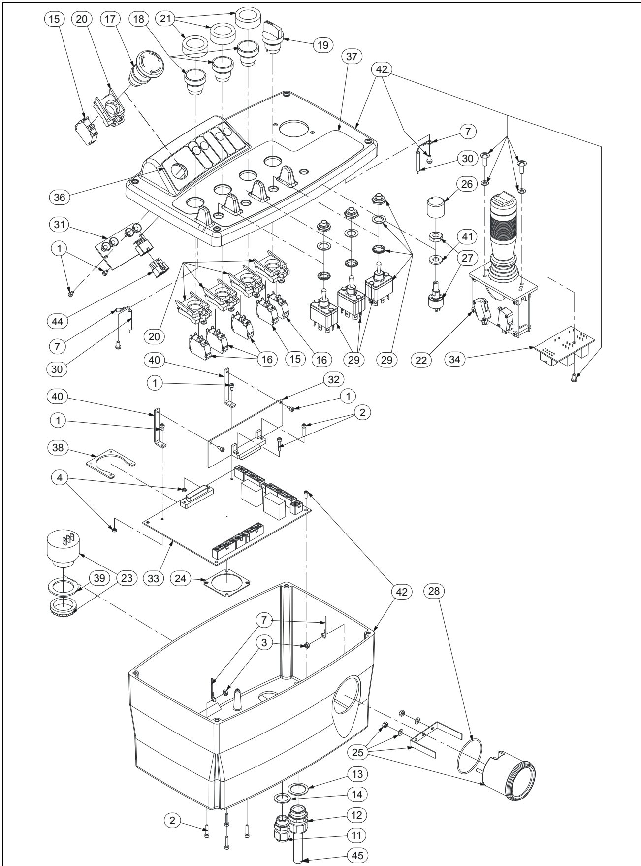
FIGURE 2-3-5.S/N SINCE / DEPUIS E18MJ #A300018047 & E26MJ #A300026073 UCB
