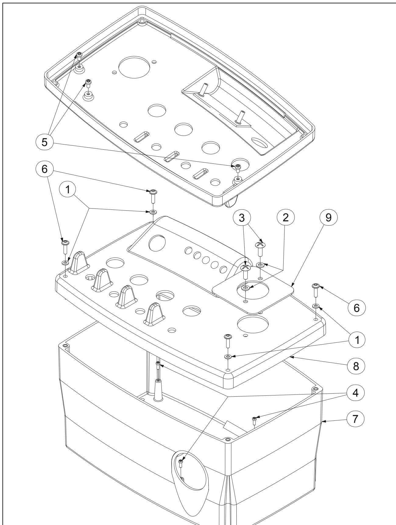
FIGURE 2-3-5-2.S/N SINCE/DEPUIS E18MJ #A300018052 & E26MJ #A30002684 PLASTIC UPPER CONTROL BOX / BOITIER HAUT PLASTIQUE
