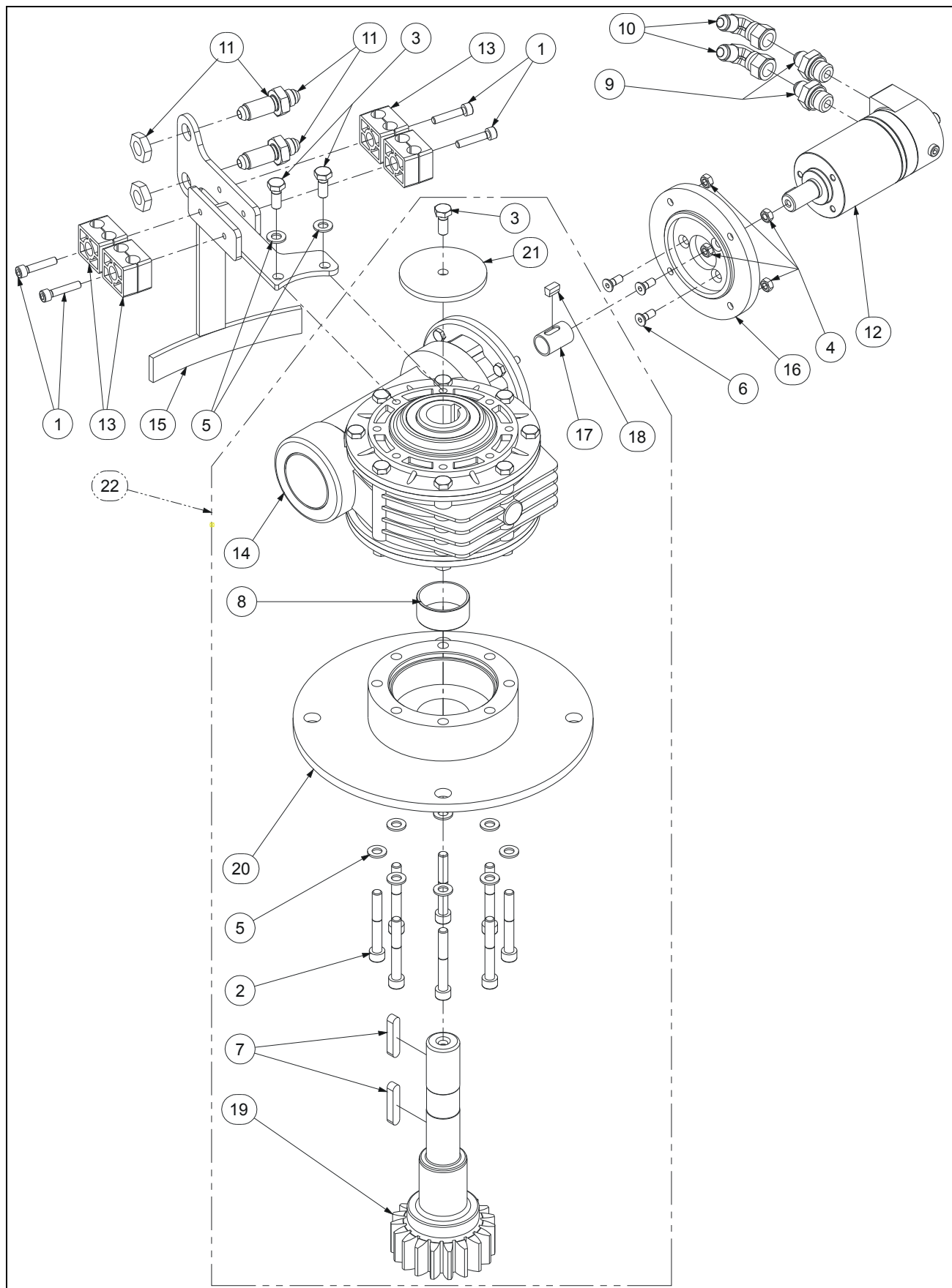
FIGURE 3-3-1. GEAR BOX ASSEMBLY / ASSEMBLAGE MOTO-REDUCTEUR
