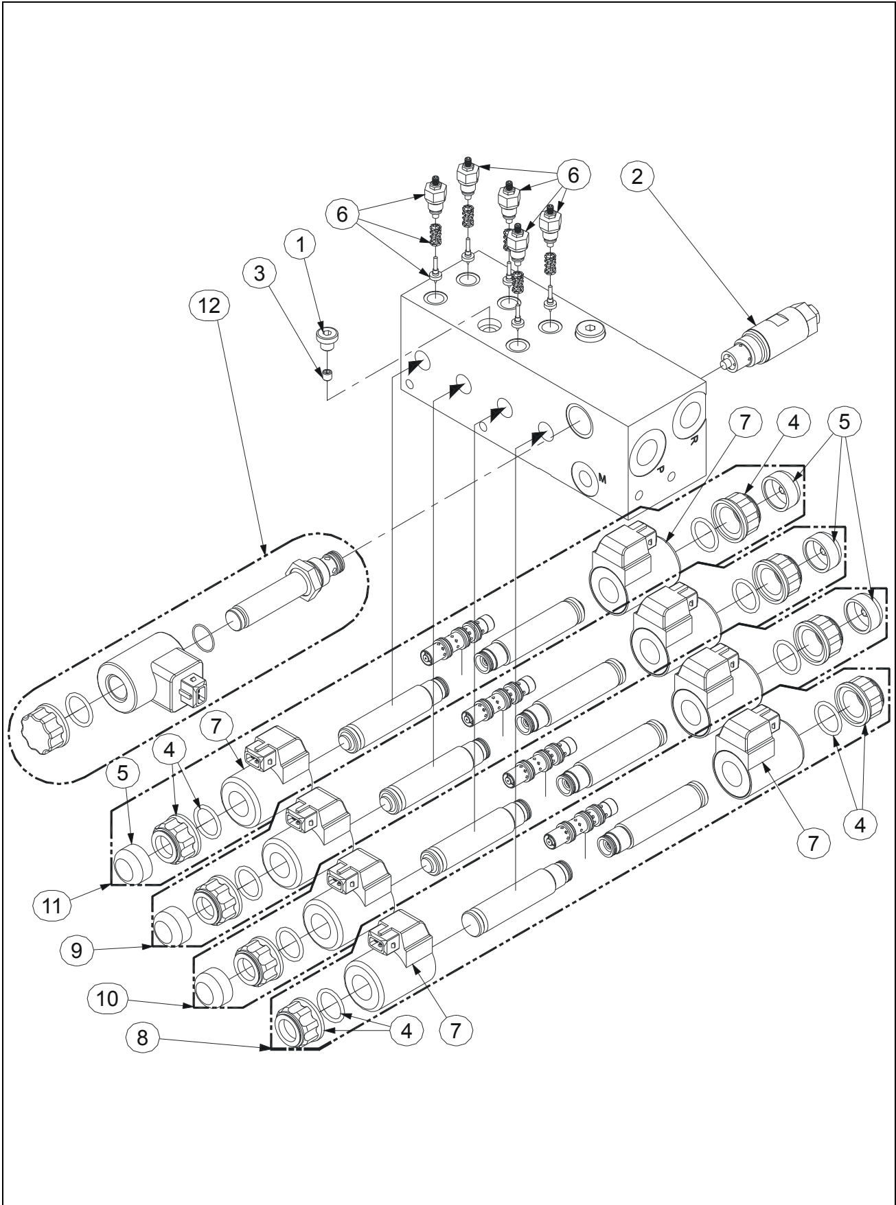
FIGURE 4-1-2-1. FUNCTIONS MANIFOLD / BLOC FONCTIONS
