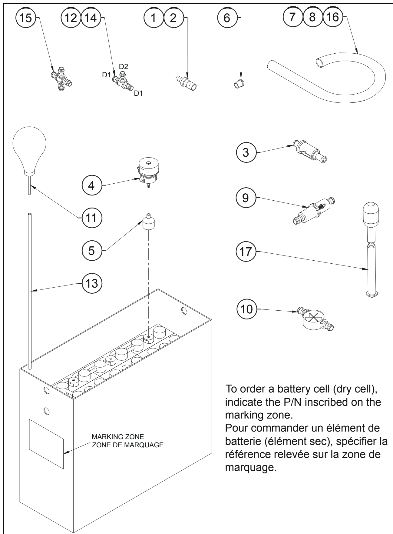
FIGURE 6-4. BATTERY COMPONENTS / COMPOSANTS BATTERIE
