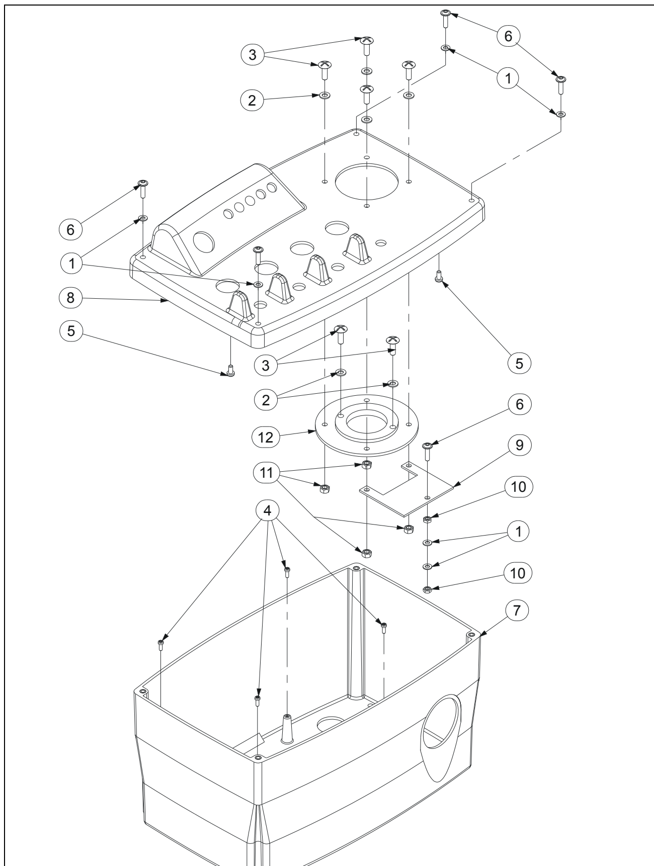
FIGURE 2-3-5-1.S/N PRIOR/AVANT E18MJ #A300018052 & E26MJ #A30002684 PLASTIC UPPER CONTROL BOX / BOITIER HAUT PLASTIQUE
