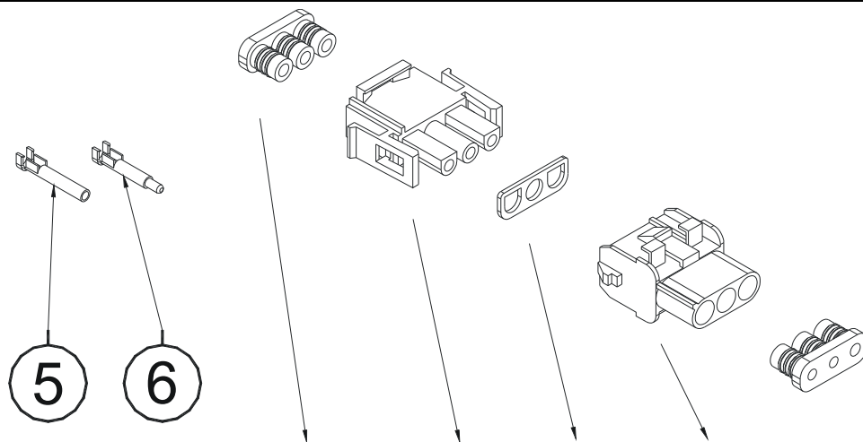
FIGURE 2-3-1.MATE-N-LOK CONNECTORS / CONNECTEURS MATE-N-LOK
