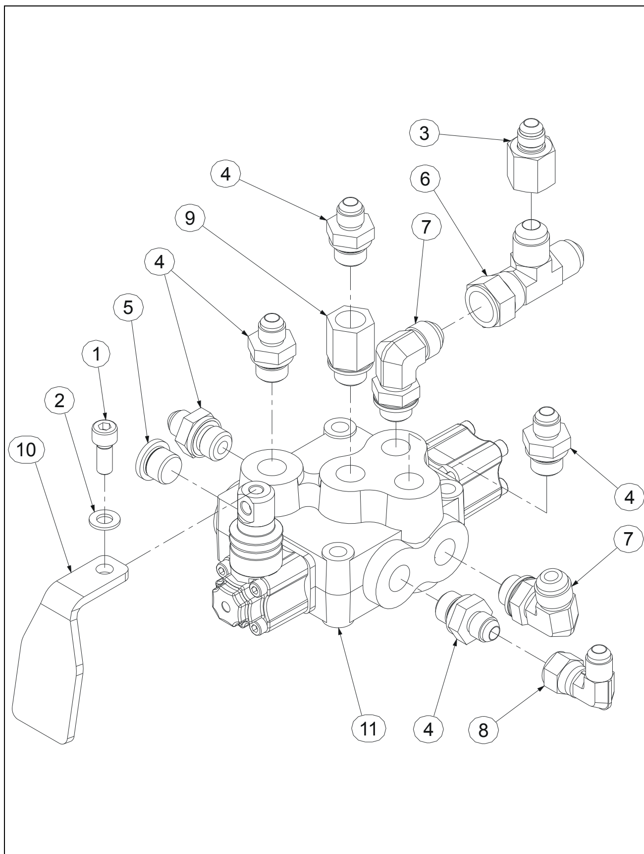
FIGURE 4-1-7. RELEASE VALVE ASSEMBLY / ASSEMBLAGE DISTRIBUTEUR DE DEBRAYAGE
