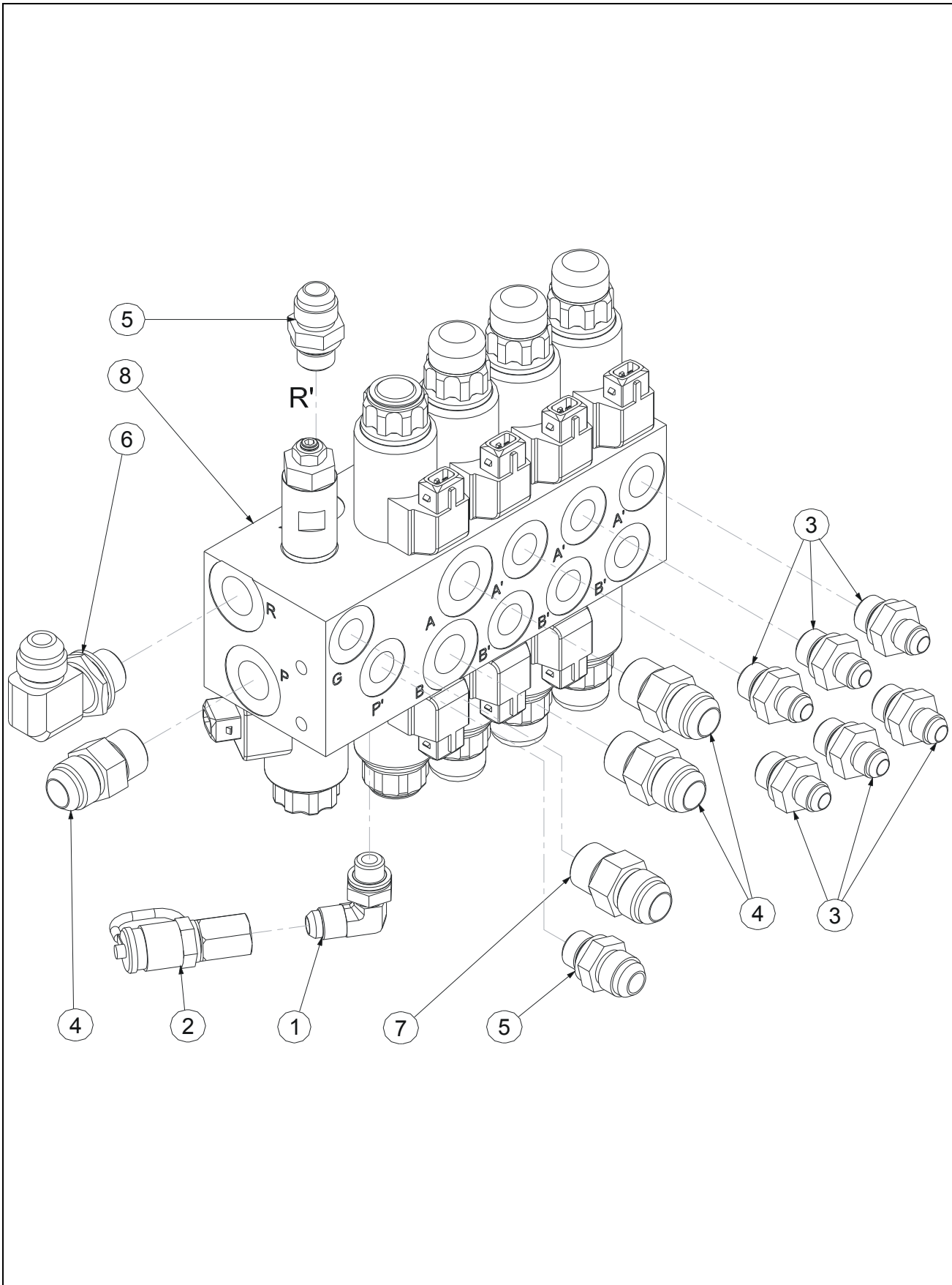
FIGURE 4-1-2. FUNCTIONS MANIFOLD ASSEMBLY/ASSEMBLAGE BLOC FONCTIONS
